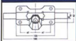
ACOTACIONES - CERROJOS A1
