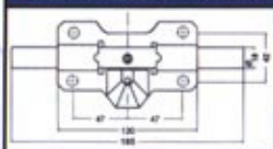
ACOTACIONES - CERROJOS B1
